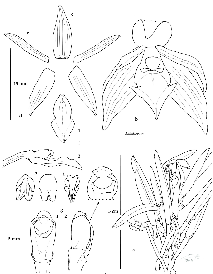
Fig. 1 : Leptotes beatricis
